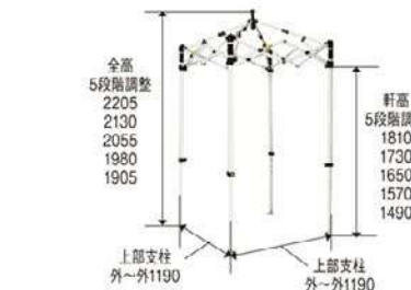
フレーム
