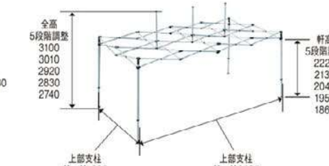
フレーム
