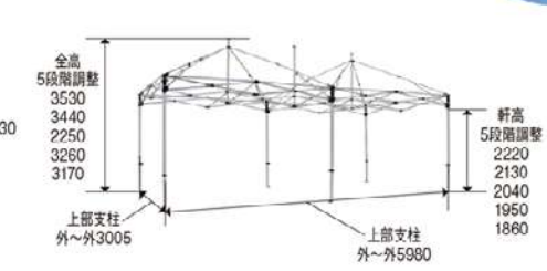
フレーム
