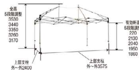
フレーム
