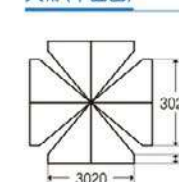
天幕(平面図)
