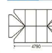
天幕(平面図)
