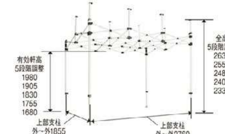
フレーム
