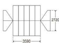
天幕(平面図)
