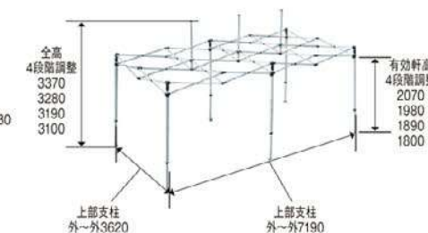
フレーム
