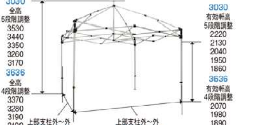
フレーム(NW/SNW共通)
