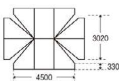
天幕(平面図)
