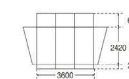
天幕(平面図)
