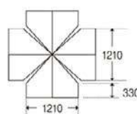
天幕(平面図)
