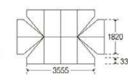
天幕(平面図)
