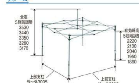
フレーム
